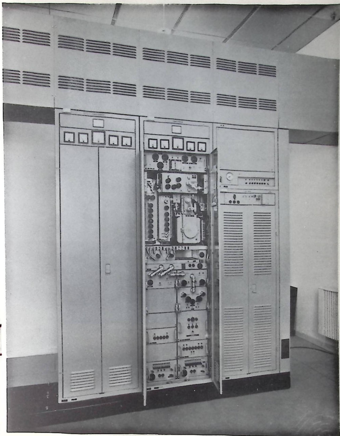
Stativ tillhörande radiolänkutrustningen
