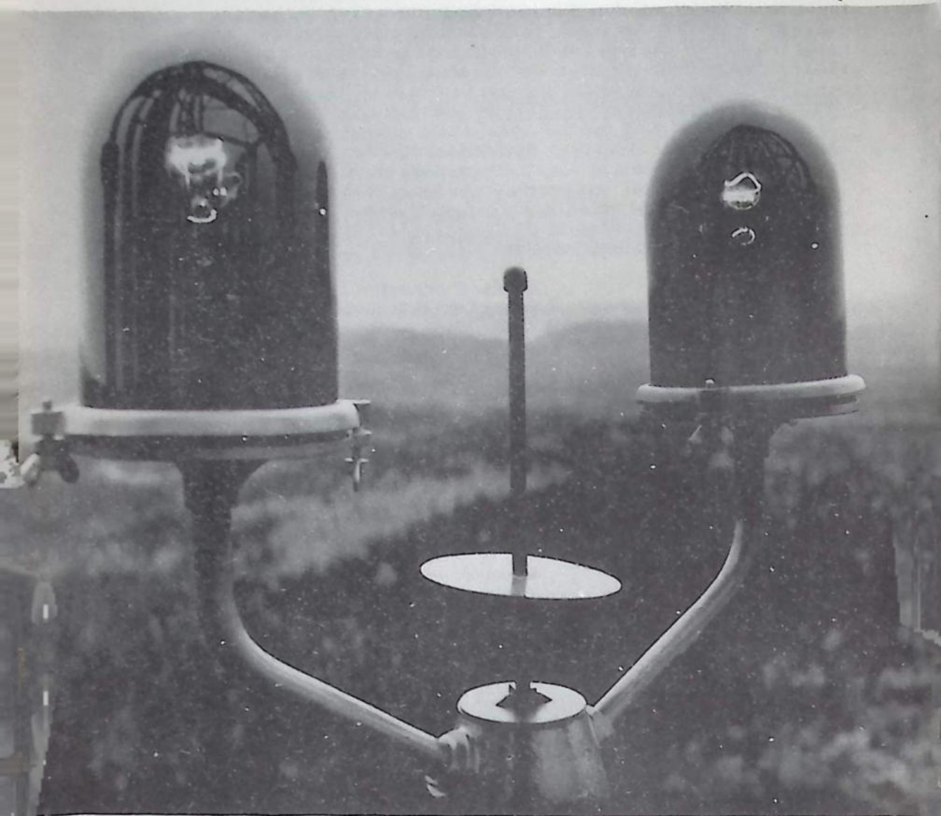
Röda hindermarkeringsljus finns på ungefär var 50:e meter i masten
