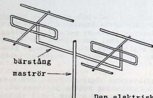
Horisontal polarisation
