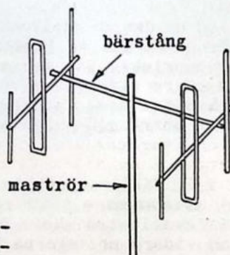
Vertikal polarisation
