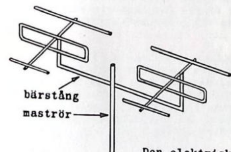
Horisontal polarisation
