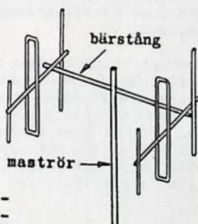
Vertikal polarisation
