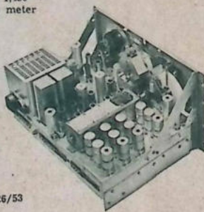
Sextonrörsradion ger ett sobert intryck — den invecklade inredningen är överskådlig.
