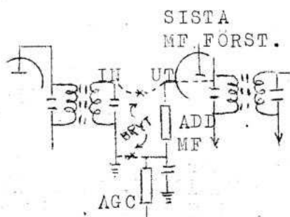
Fig.1 - Inkoppling i mottagaren
