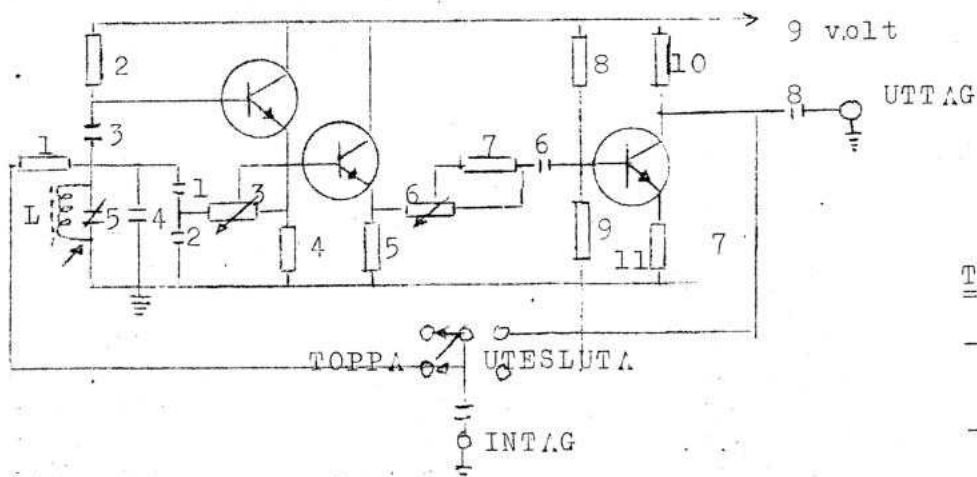
Fig.3. - komplett ritning till Q-multipliern
