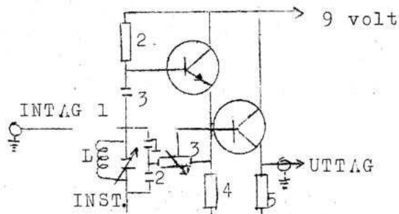
Fig.2 - grundläggande uppfattning om Q-multipliern
