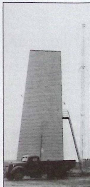
Kyltorn, och en av masterna 1952 ute vid Göteborgs rundradiostation vid Järnbrott i Västra Frölunda.
