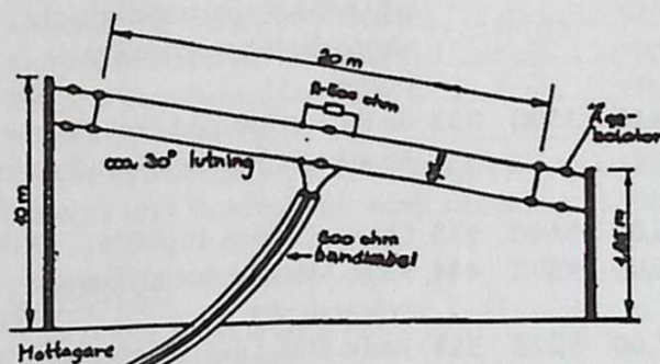
Figur 4. Bredbandig lutande dipol
