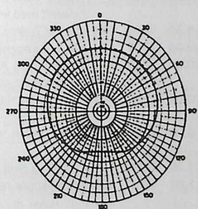
Figur 3. Horisontella strålningsdiagram
