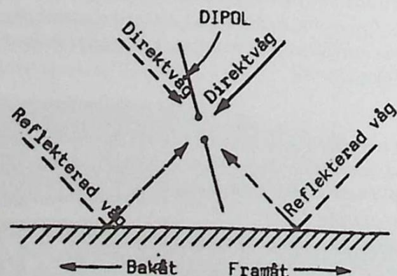
Figur 1. Lutande dipol med radiovågor
