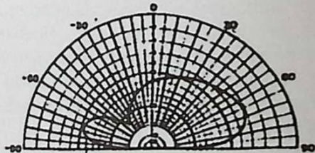
Figur2. Vertikala strålningsskärmar
