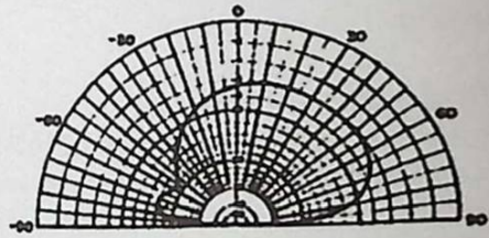
b. Lutning 45 grader
