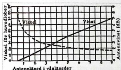
Figur 3. Vinkel och antennvinst för long-wire
