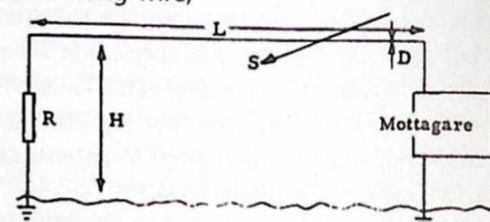
Figur 1. Principskiss över Beverageantenn
