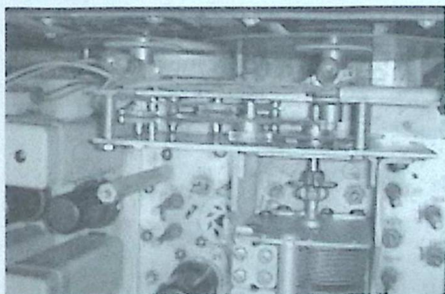
Skalorna, svänghjulet och de förspända kugghjulen i avstämningsmekanismen.
