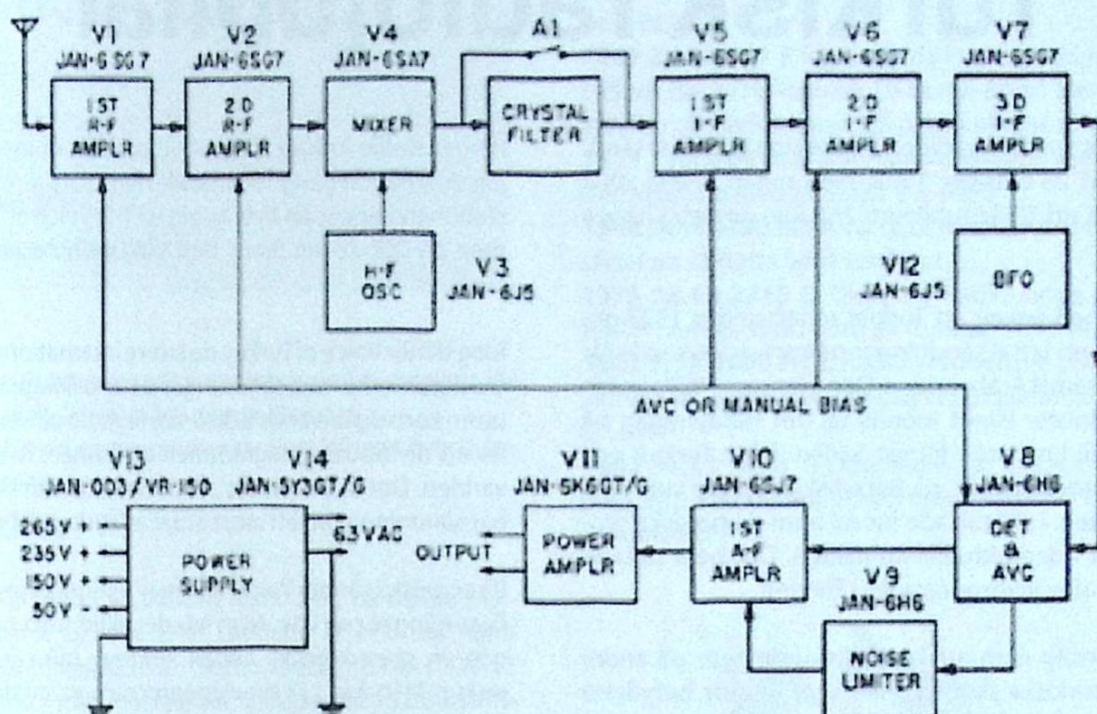
Blockschema för AR88
