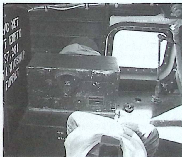
Radiooperatörens plats i B24 "Witchcraft" med en BC-348 och en J37 telegrafnyckel.
