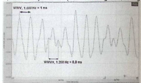
Figur 10: Denna "svävning" uppstår genom det rytmiskt olika sammanträffandet mellan "toppar" och "dalar" i de båda signaler, vilket visas här.
