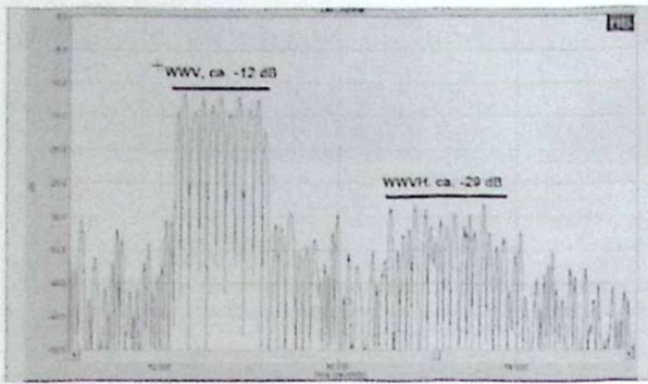
Figur 7: Vid samma AF-inställningar skiljer sig signalstyrkan mellan WWV och WWVH ca 17 dB.
