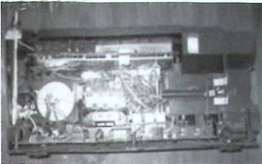
Satellit 600 med bakstycket lossat. För att komma åt att byta lampor måste man dessutom lossa framstycket och för att göra detta måste alla rattar demonteras.
