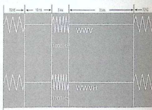
Figur 4: Varje sekundimpuls är 5 millisekunder lång. WWV och WWVH skiljer sig härvidlag i tonhöjd.
