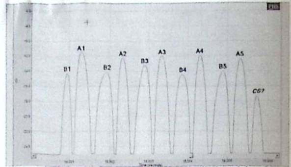
Figur 8: En sändare - två vägar. Man kan tydligt skilja på "Serie A" och "Serie B".
