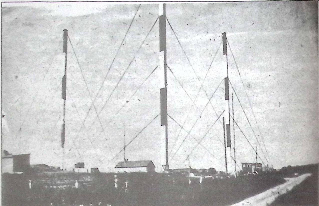
Triangelantennen uppmonterad i Hellerud utanför Oslo för Königsberggradions sista sändningar i maj 1945!
