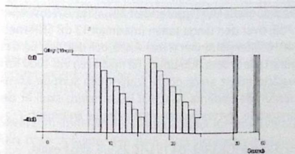
Figur 2: Sändningsschema för fyrarna med CW-id, två gånger nio toner med 6 dB effektsänkning mellan varje ton, den tio millisekunder långa 10W-tonen och de två 0,5 millisekunder breda impulserna under 30 sekunder.
