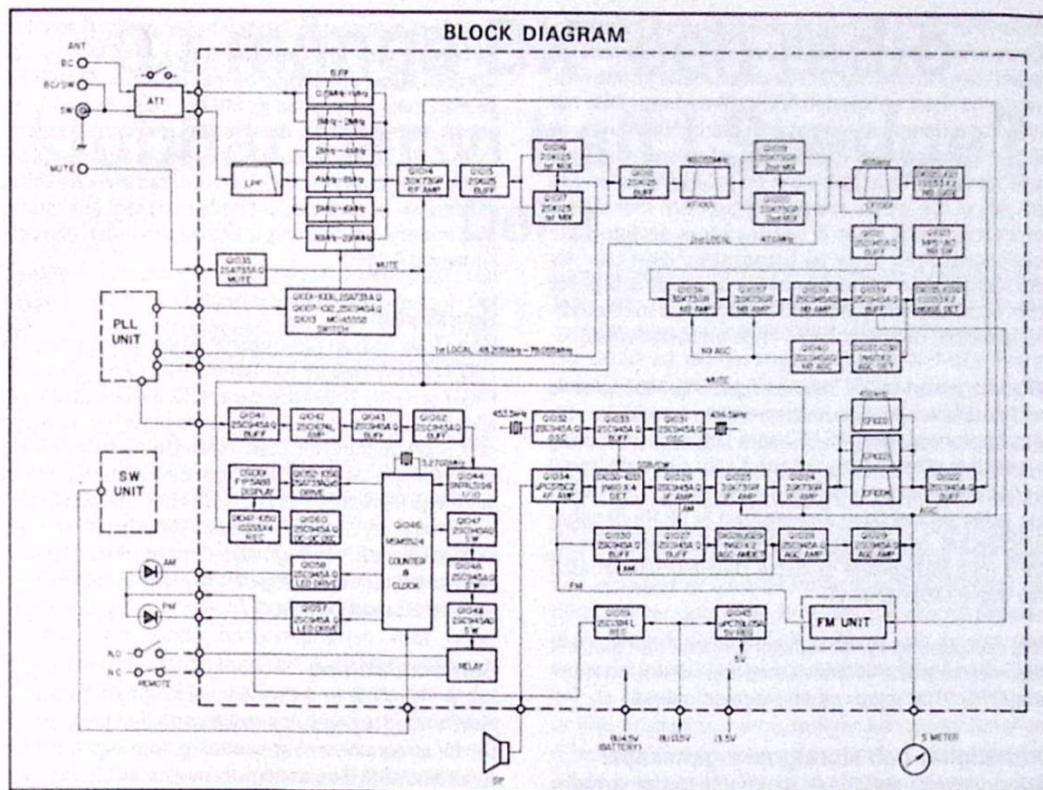
Blockdiagram för FRG-7700.
