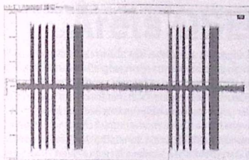
Bild 7: Var 6,5:e sekund sänder NDB 320-HA sin identifikation HA på morse - fyra punkter (H), punkt-streck (A) [14]
