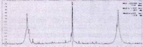
Bild 2: Den med 1 022 Hz modulerade signalen från 320-HA under frekvensluppen.
